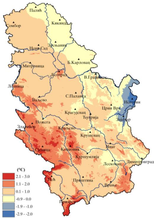
Слика 1. Одступање средње температуре ваздуха од нормале 1991–2020. године за период 18–24.10.2024. године
