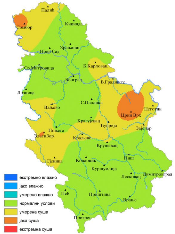
Слика 4. Прогноза Стандардизованог падавинског индекса одређеног за временски период од 60 дана (SPI-2) рађена на основу осматраних (5.10–24.10.2024 године) и прогнозираних падавина (25.10–3.11.2024. године) Европског центра за средњорочну прогнозу времена и Републичког хидрометеоролошког завода
